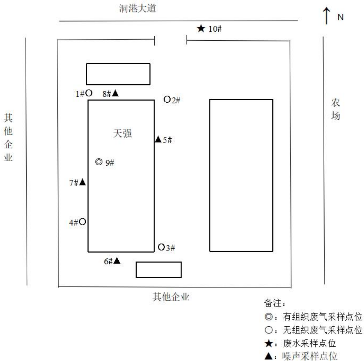
附图3 厂区平面布置及采样点位示意图
