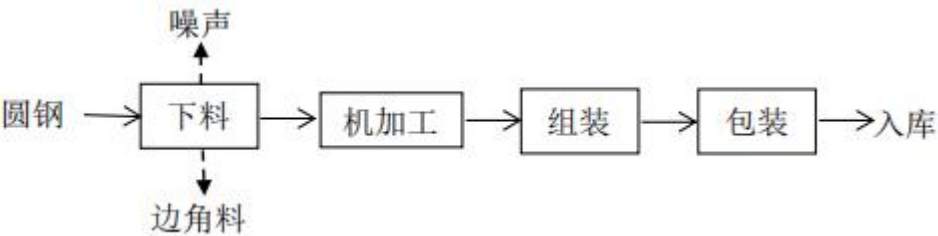
图2-3启动阀生产工艺流程及产污环节图
