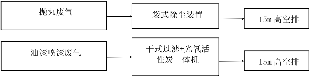
图 3-2 实际废气处理流程图
