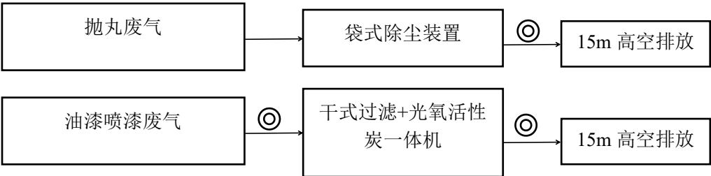
图6-2 废气采样点位示意图
