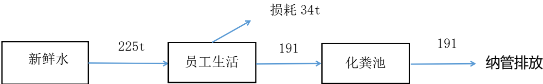
图2-1项目水平衡图
