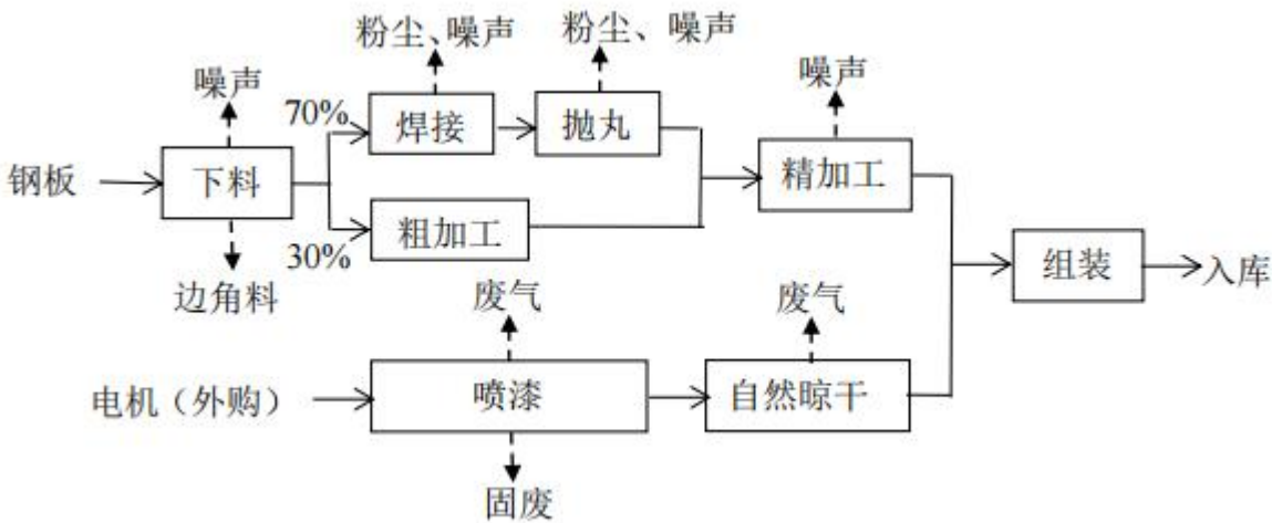
图2-2鼓风机生产工艺流程及产污环节图
