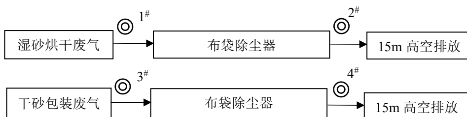
图 6-2 有组织废气采样点位示意图
