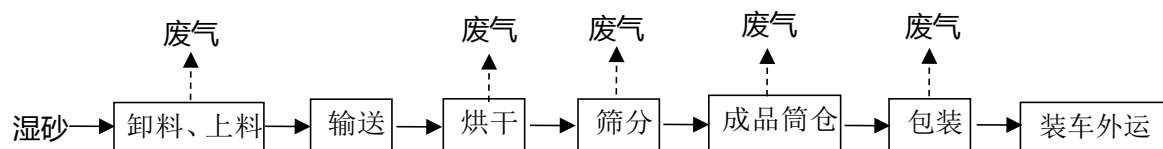
图2-2 干砂生产工艺流程图
